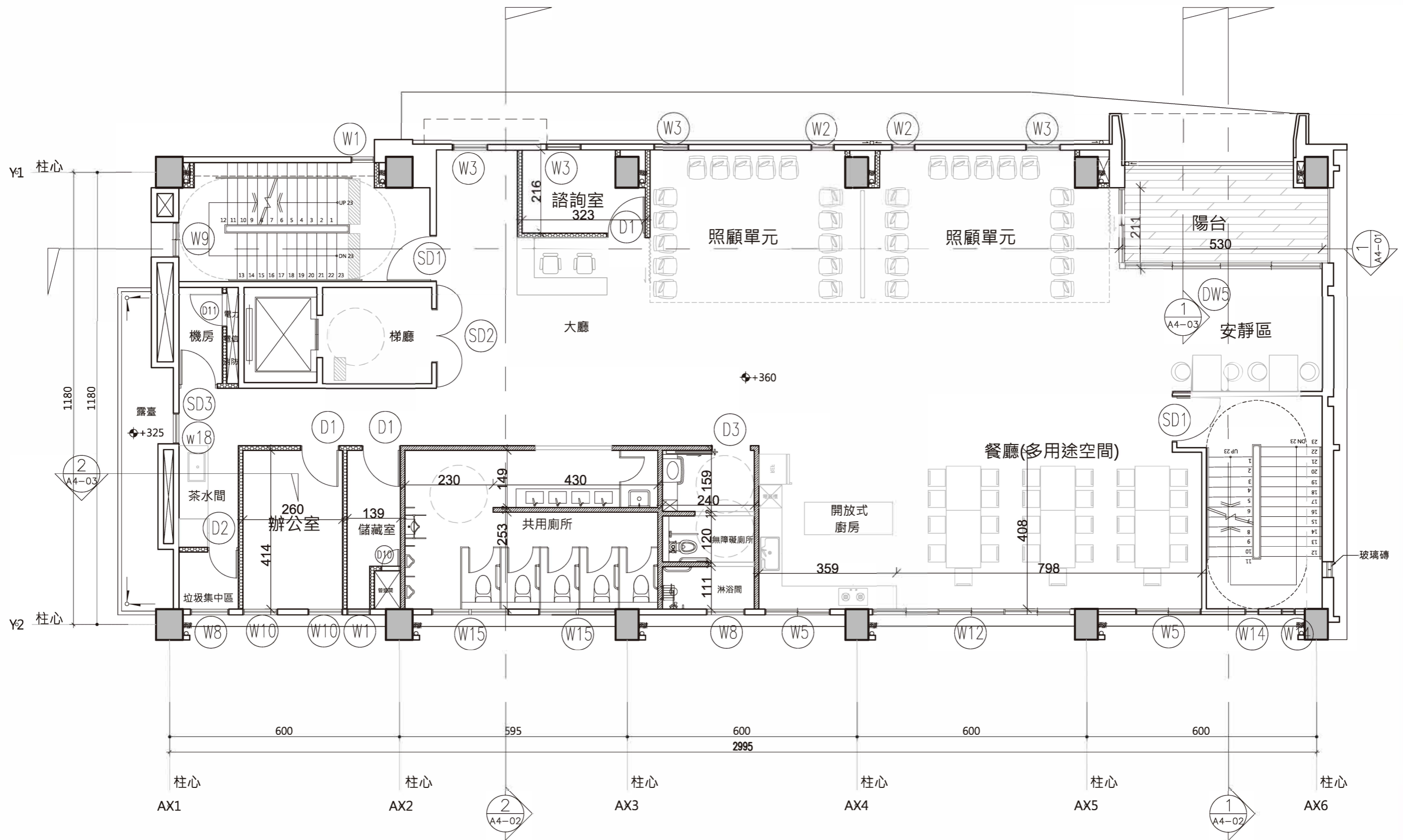
1 二層平面圖 S:1/100(A3) 1/50(A1)
